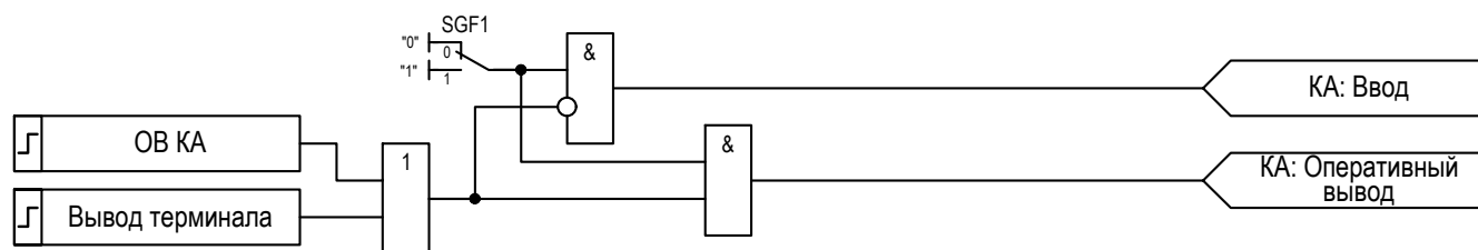
Рисунок 2.19 – Логика управления режимами функционального блока «КА»
