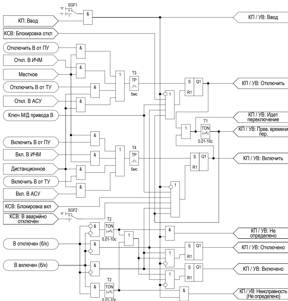
Рисунок 2.18 – Функциональная схема «УВ»
