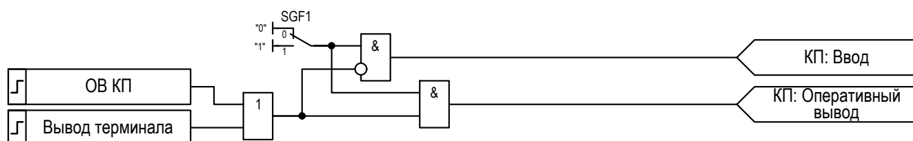
Рисунок 2.17 – Функциональная схема управления режимами работы «КП»
